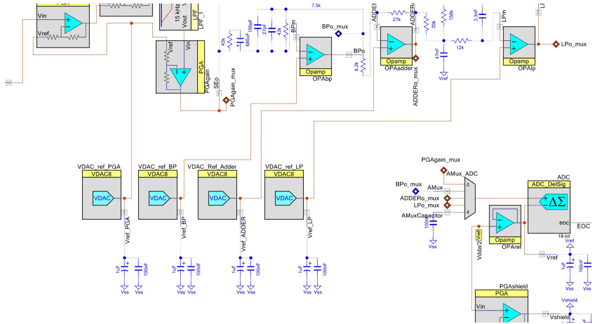
Figura 2: Cadena de acondicionamiento consolidada en PSoC Creator. El recorte comienza después de los terminales de entrada para mantener esta sección independiente del transductor: PGA diferencial, ganancia adicional, MFB, sumador, LP, referencias independientes, AMux y ADC. La captura corresponde a la revisión histórica con VDAC.
