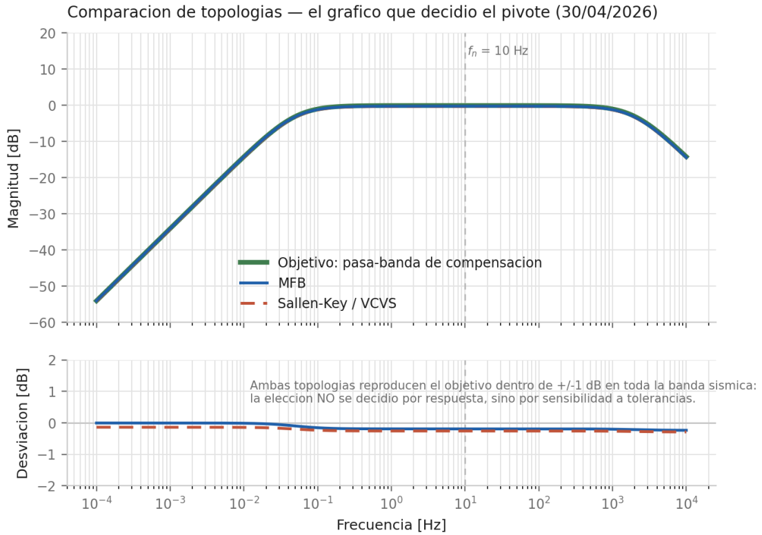
Figura 1: Comparación reconstruida a partir del análisis utilizado el 30 de abril. La magnitud nominal no decide el pivote: el criterio principal es la robustez frente a tolerancias al replicar canales.
